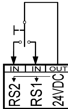
Afb.6 Starten op afstand
