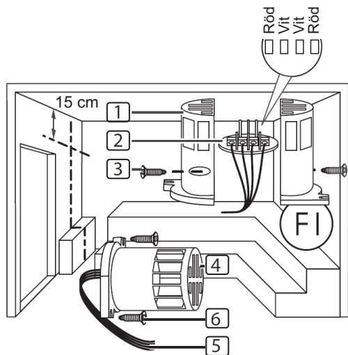
Bild 5 Montering av ugnsgivare
