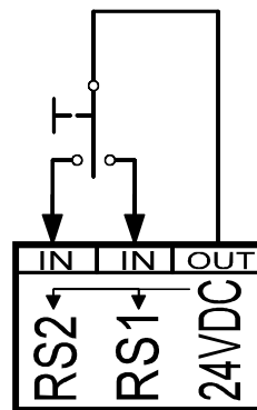
Abb.6 Fernstart
